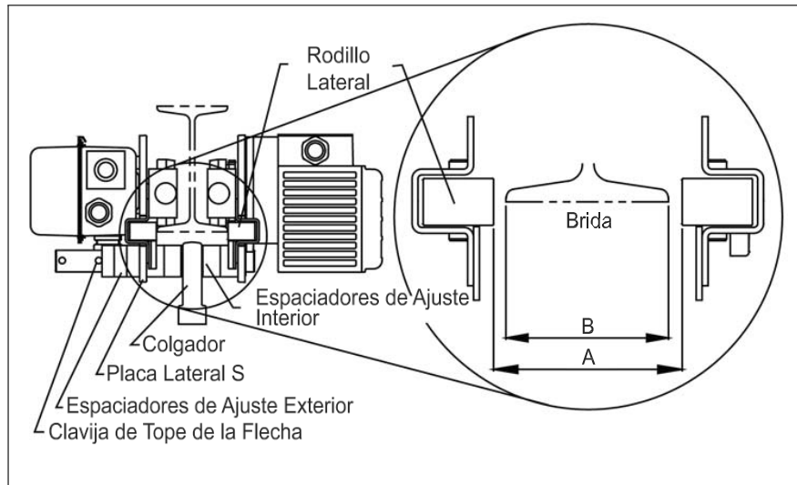
Figura 3-8 Ajuste del trole – Hasta de 5 toneladas de capacidad
