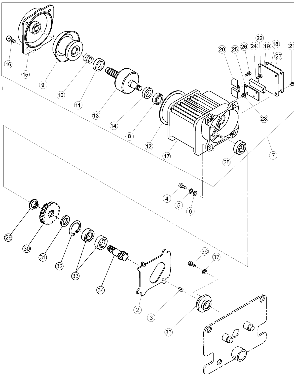
Figura 9-6 Partes del Motor
