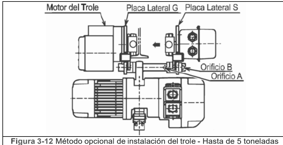
Figura 3-12 Método opcional de instalación del trole - Hasta de 5 toneladas
