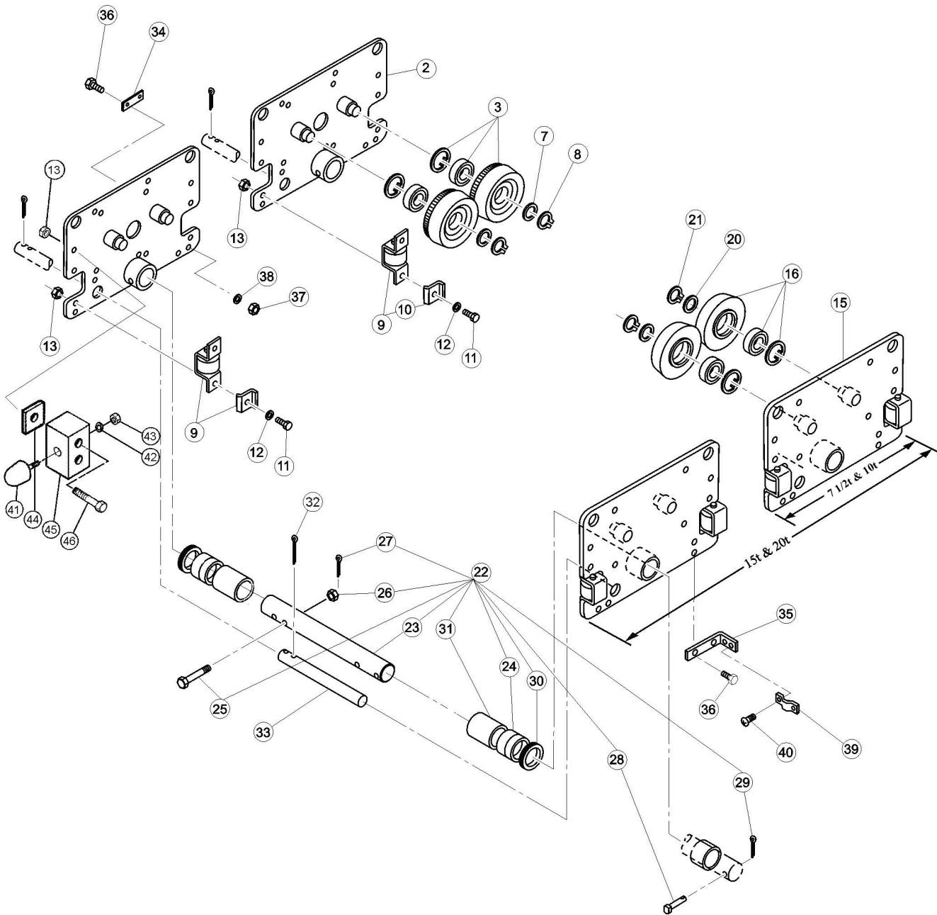
Figura 9-7 Placas Laterales y Partes de Suspensión
