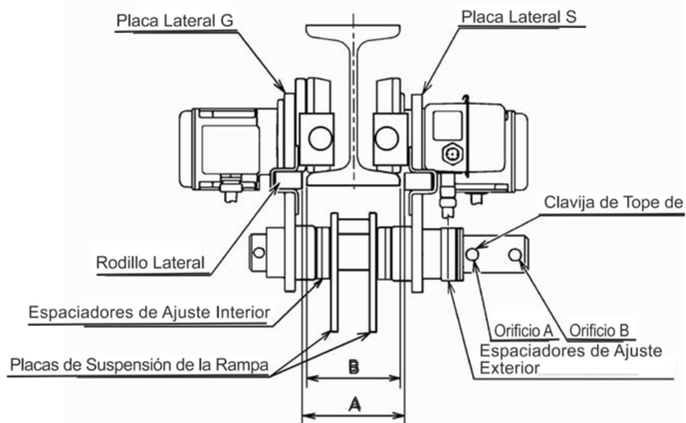
Figura 3-9 Ajuste del trole – De 7.5 a 20 toneladas de capacidad
