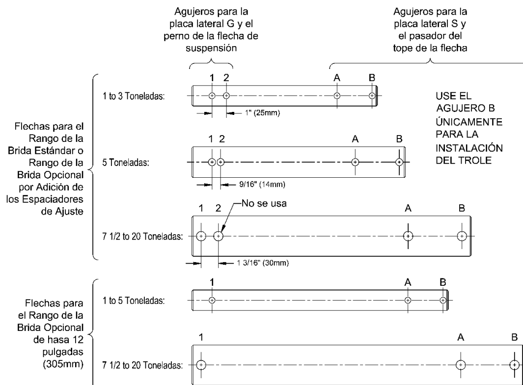
Figura 3-7 Flechas de suspensión
