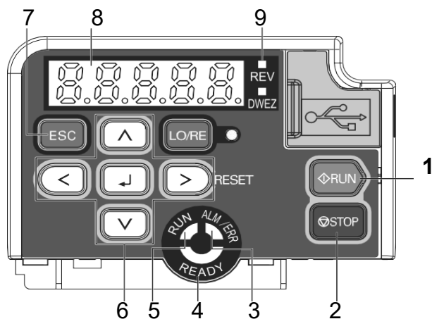
Figura 3-18 (cont.) Interfaz de teclado/pantalla para variador de frecuencia (VFD) MR2B – Solo modelos MR2B (VFD de nuevo diseño); consulte la tabla 3-3 a continuación
