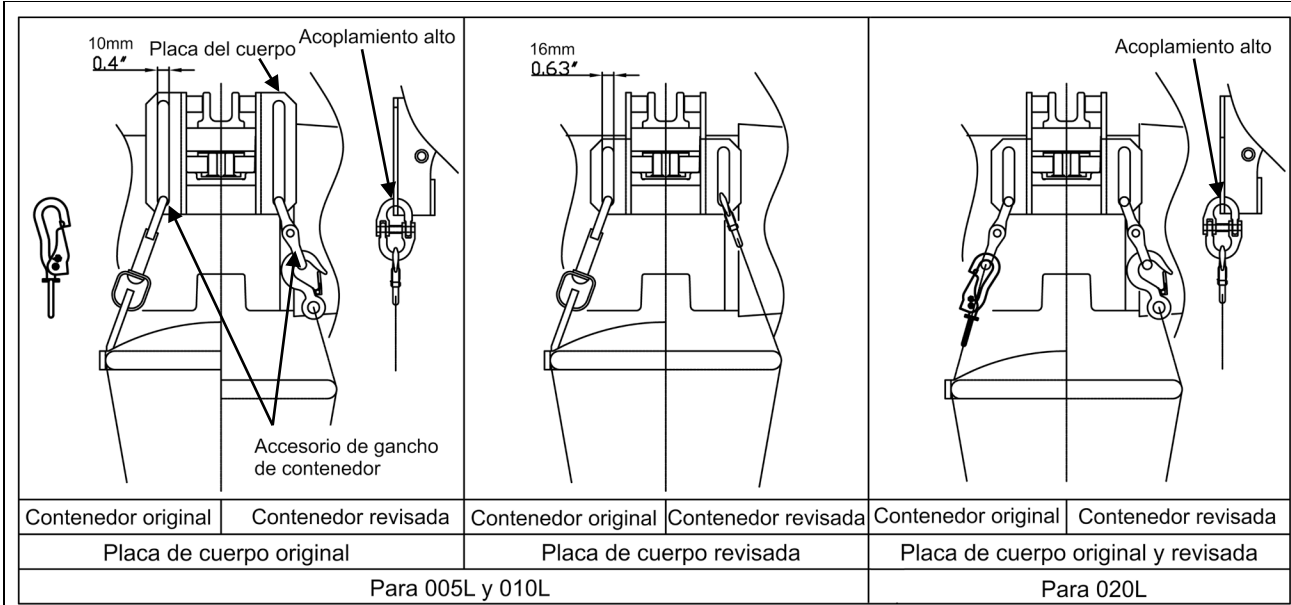
Figura 3-2 Fijación del recipiente de cadena al cuerpo del polipasto/tecle
