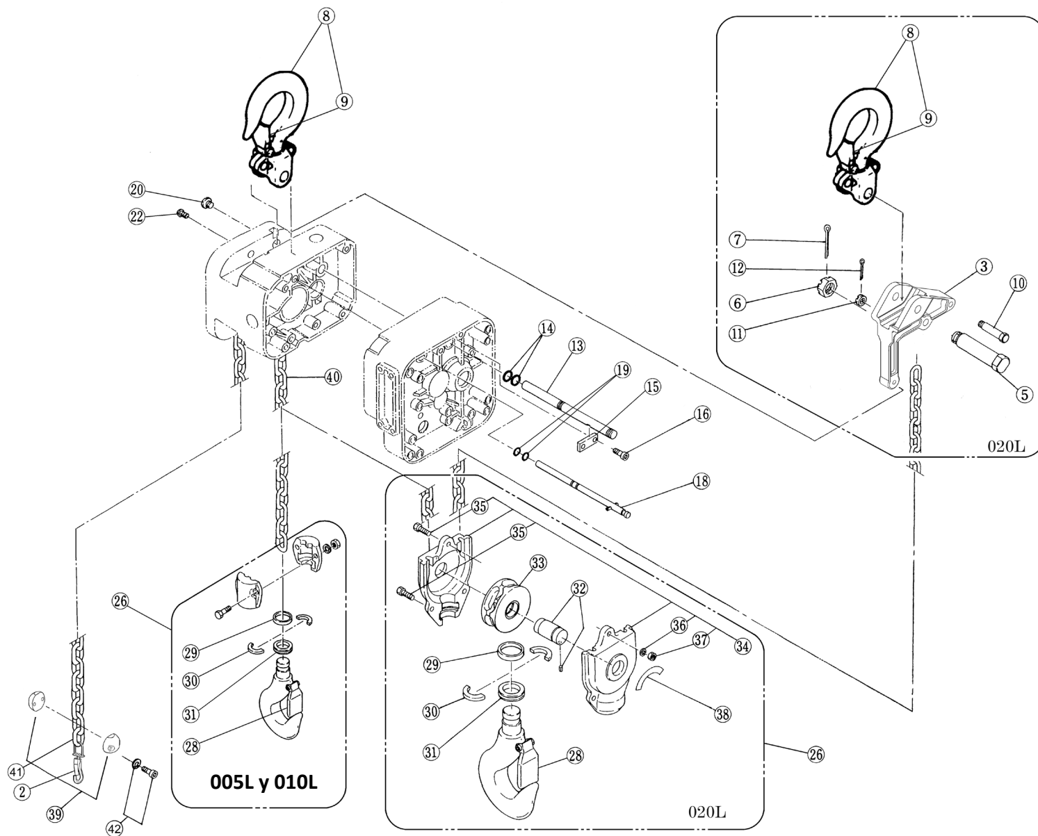
Figure 9-3 Piezas del gancho
