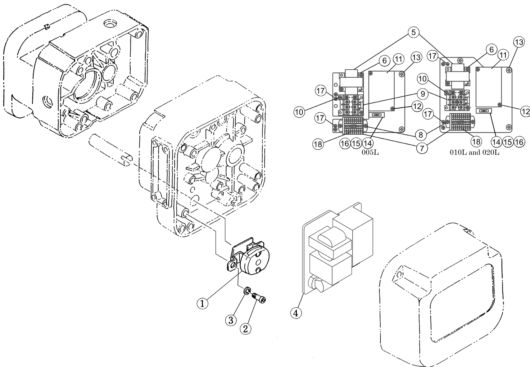
Figure 9-5 Piezas eléctricas
