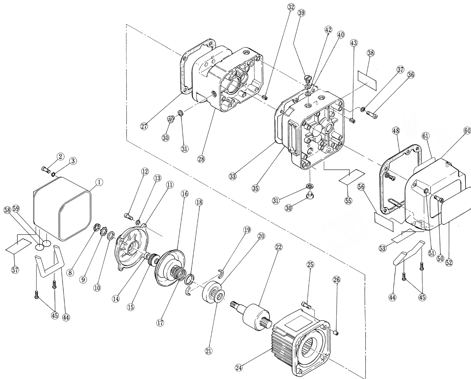
Figura 9-1 Piezas del motor y de la carcasa
