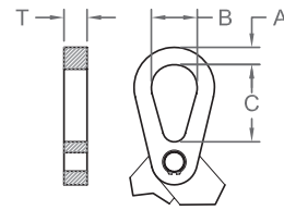
Opción de suspensor UBC
