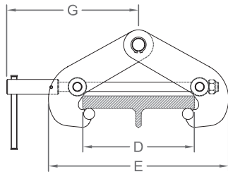
Abrazadera universal de viga
